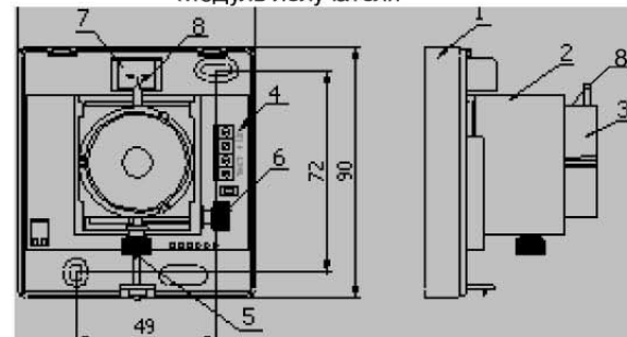
Модуль излучателя
