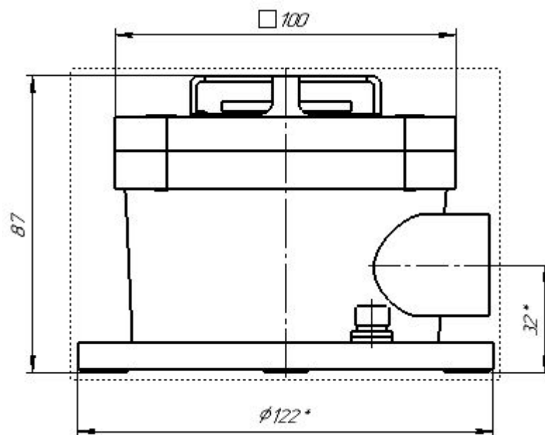
Рис А. Габаритные размеры дымового точечного извещателя Спектрон-ДИП-31-Exd-A/Н
