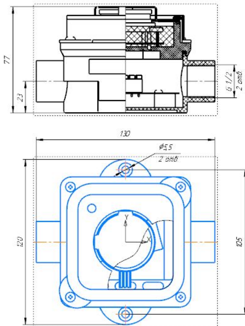
Рис А. Габаритные размеры дымового точечного извещателя Спектрон-ДИП-31-Exi/Exm
