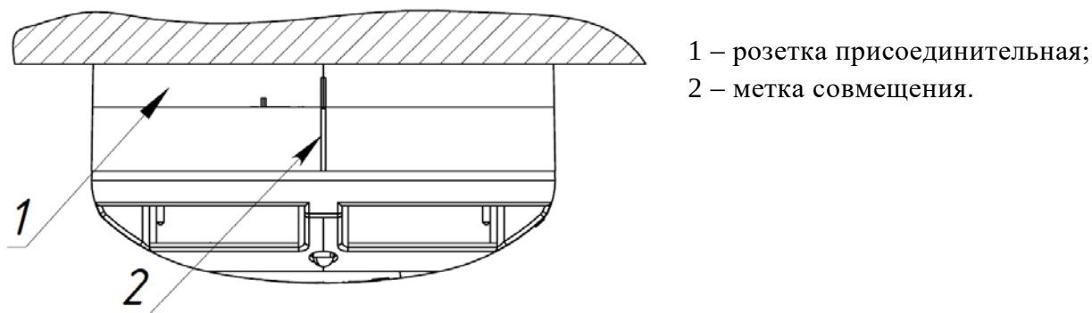
Рисунок 2.2.3.1 Установка извещателя
