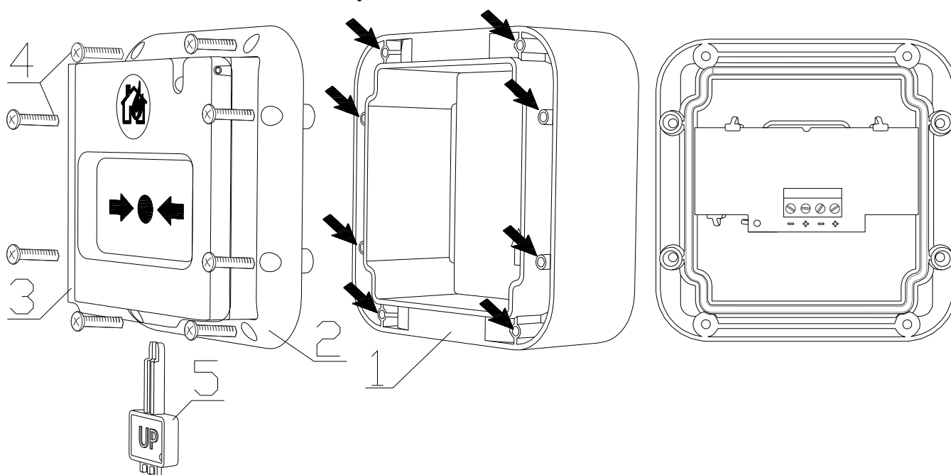
Рисунок 2.2.3.1 Основание ИПР
