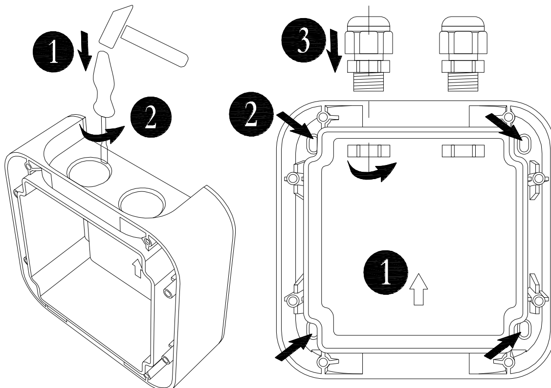
Рисунок 2.2.3.1 Основание ИПР
