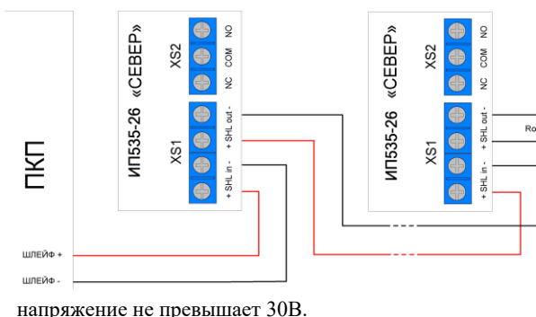
Рис.2. Схема подключения извещателей в шлейф
