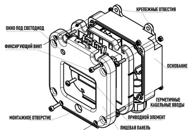
Рис.1. Элементы конструкции извещателя
