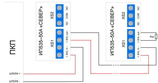
Рис.2. Схема подключения извещателей в шлейф
