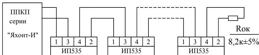
Рис.8.1 Схема подключения извещателей ИП535 к приборам серии «Яхонт И»
