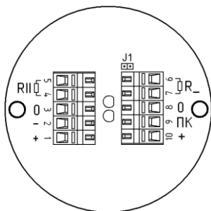
Рисунок 4. Внешний вид платы извещателя ИП5335-07е.
