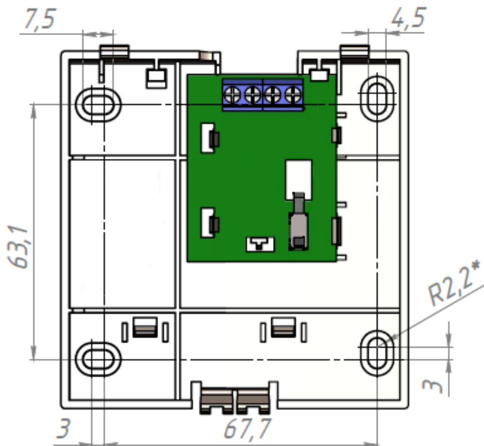
Рисунок 2.2.2.2 Установочные размеры ИПР
