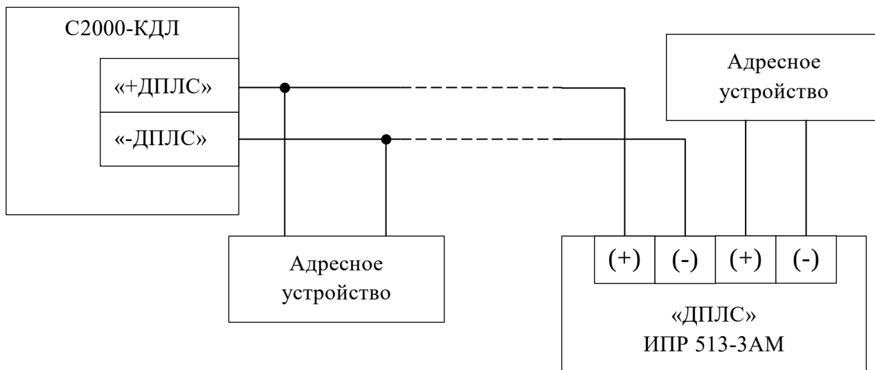
Рисунок 2.2.4.1 Схема внешних соединений
