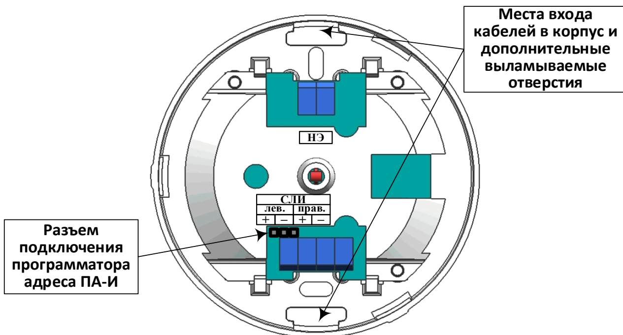
Рисунок 102 – Клеммы подключения внешних цепей к ИПТ-СИ-л, ИПТ-И-л, МКС-И-л.
