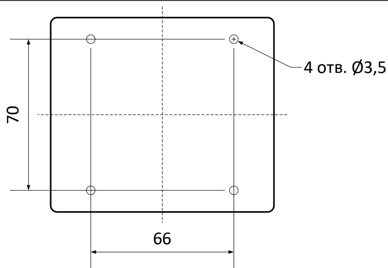
Рисунок 130 – Установочные размеры модулей.
