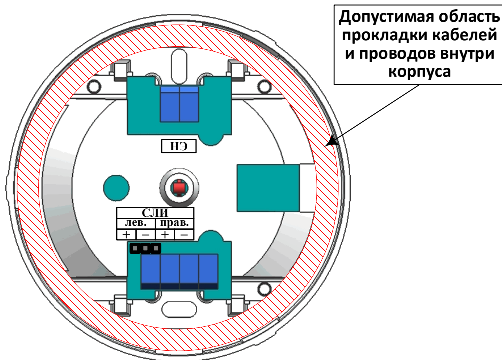
Рисунок 103 – Области прокладки кабелей (проводов) внутри ИПТ-СИ-л, ИПТ-И-л, МКС-И-л.
