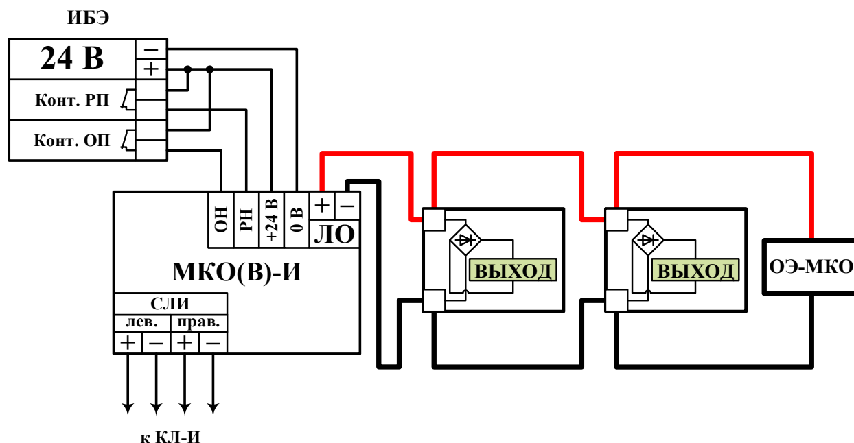
Рисунок 125 – Схема подключения оповещателей к МКО(В)-И. ИБЭ с релейными выходами исправности входов электроснабжения.
