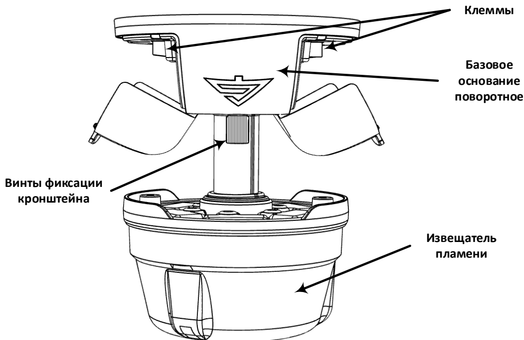
Рисунок 113 – Внешний вид ИПП-СИ.
