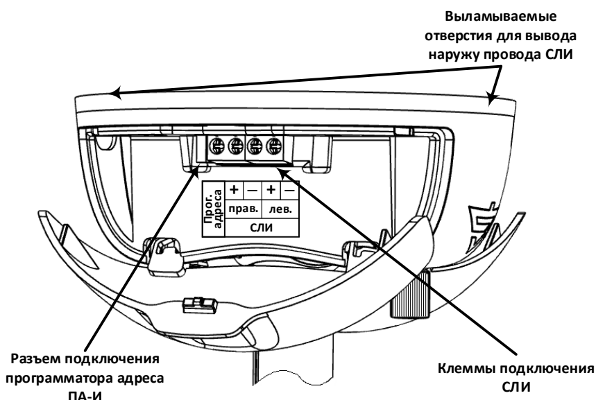
Рисунок 117 – Подключение СЛИ.
