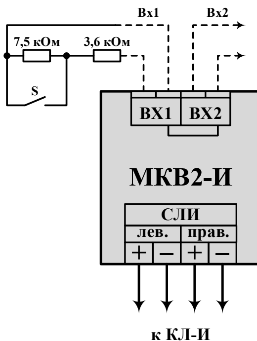
Рисунок 128 – Схема подключения внешних цепей к модулям контроля входов на примере МКВ2-И.
