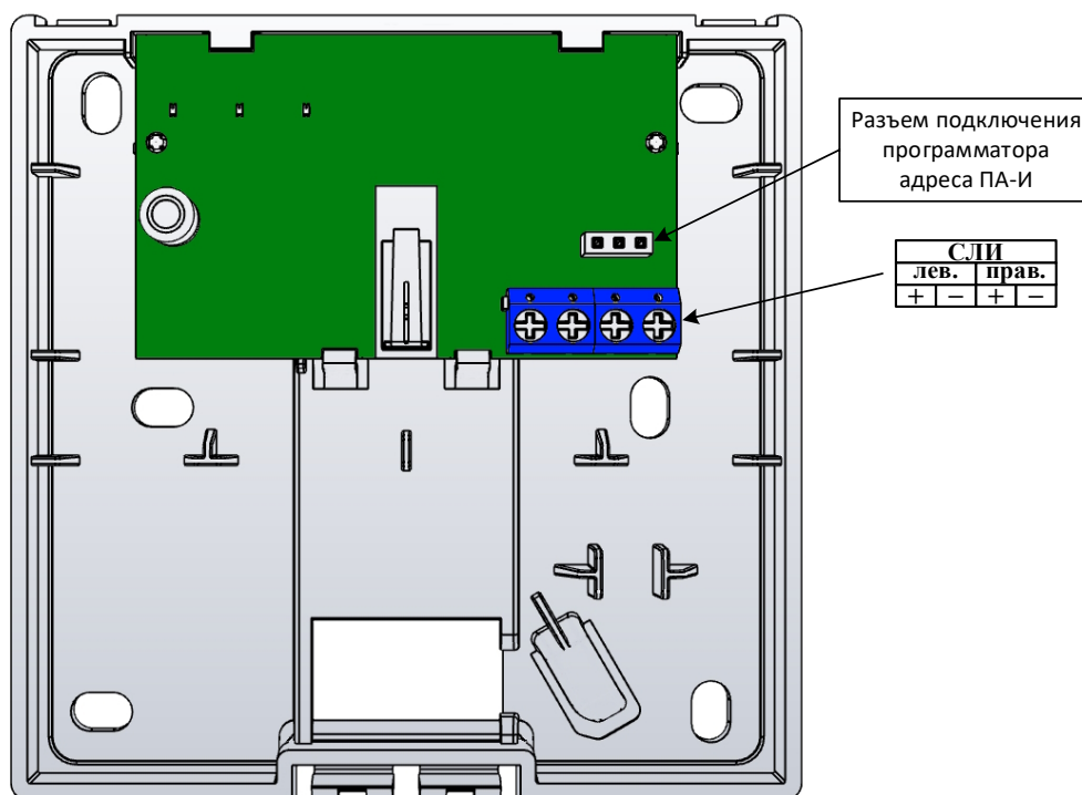
Рисунок 119 – Клеммы подключения внешних цепей к ИПР-И.
