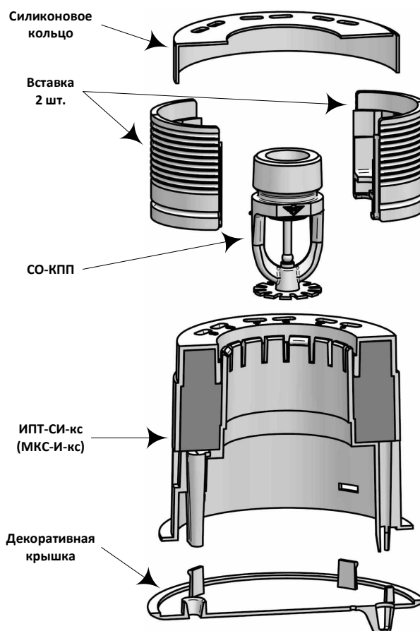
Рисунок 110 – Схема установки ИПТ-СИ-КС и МКС-И-КС на СО-КПП.
