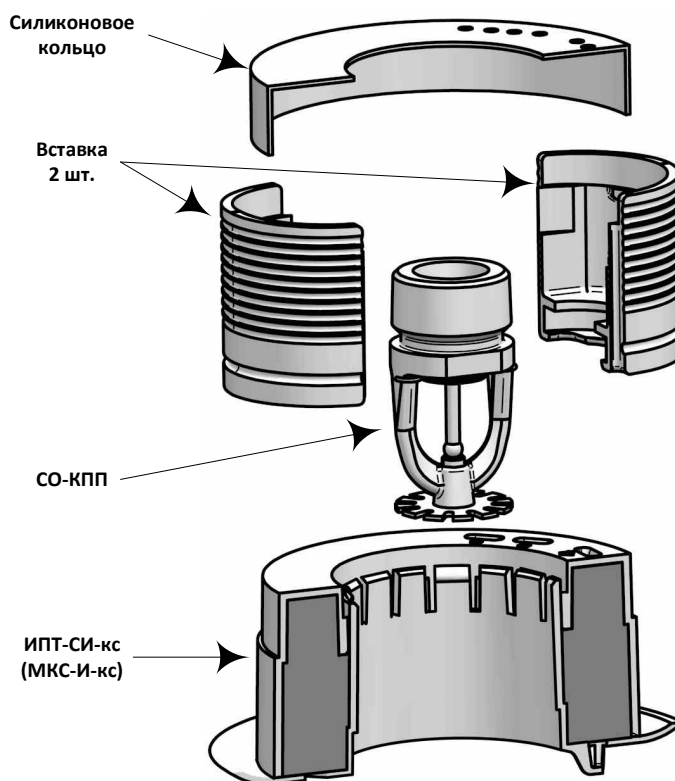
Рисунок 109 – Схема установки ИПТ-СИ-ку и МКС-И-ку на СО-КПП.
