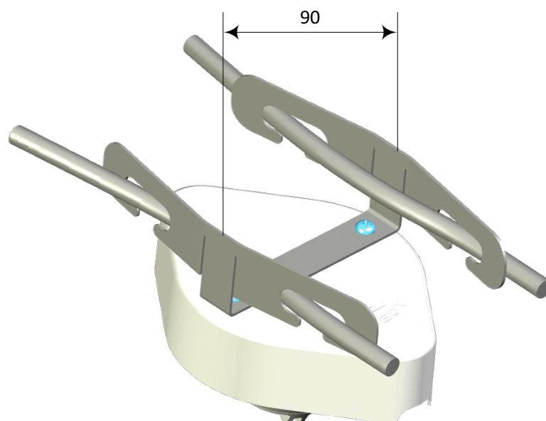
Рисунок 108 – Кронштейн крепления тросовый.
