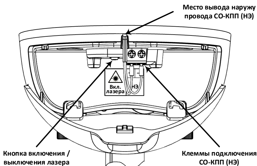
Рисунок 116 – Подключение НЭ СО-КПП.
