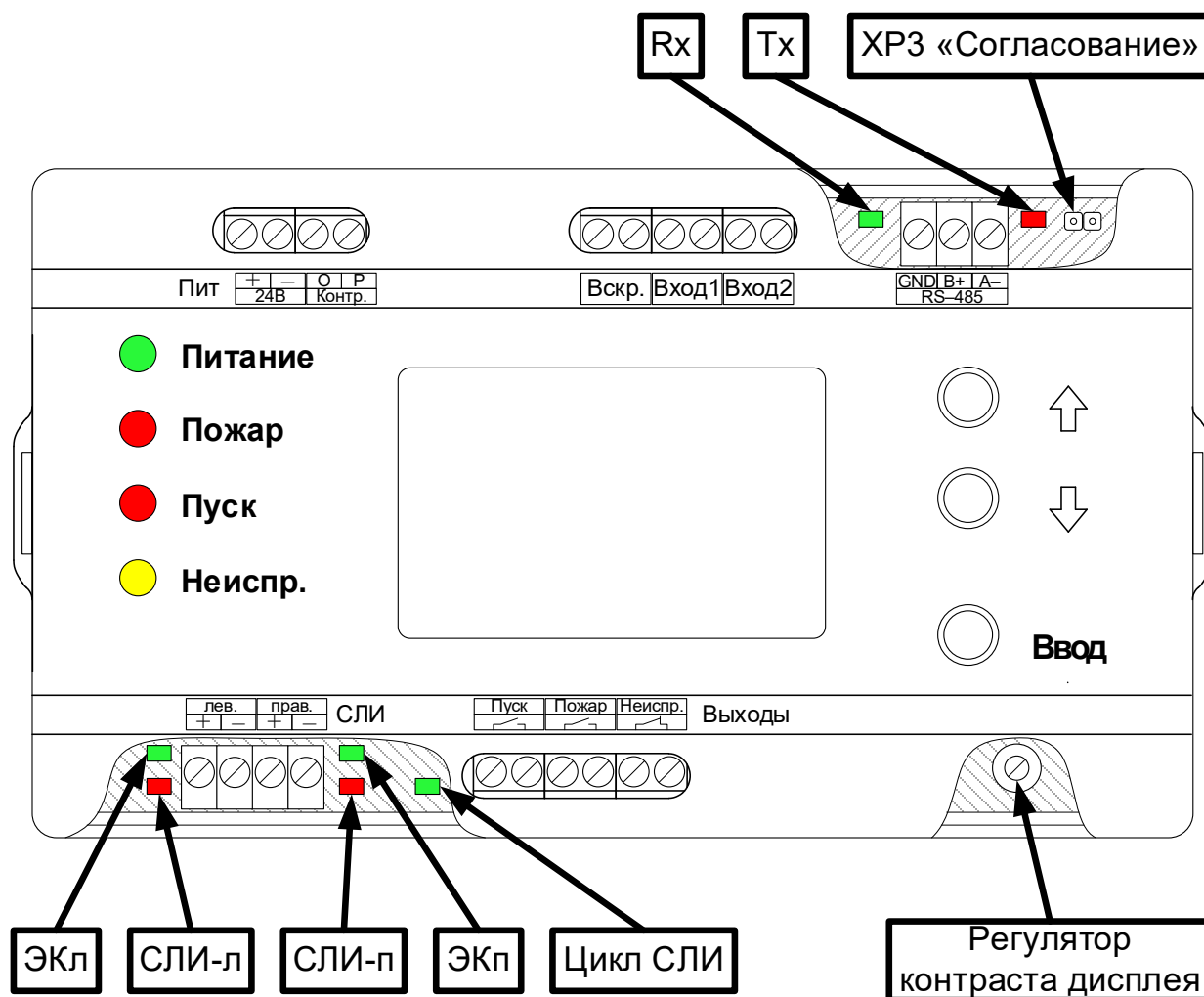
Рисунок 25 – Внешний вид модуля КЛ-Им.
