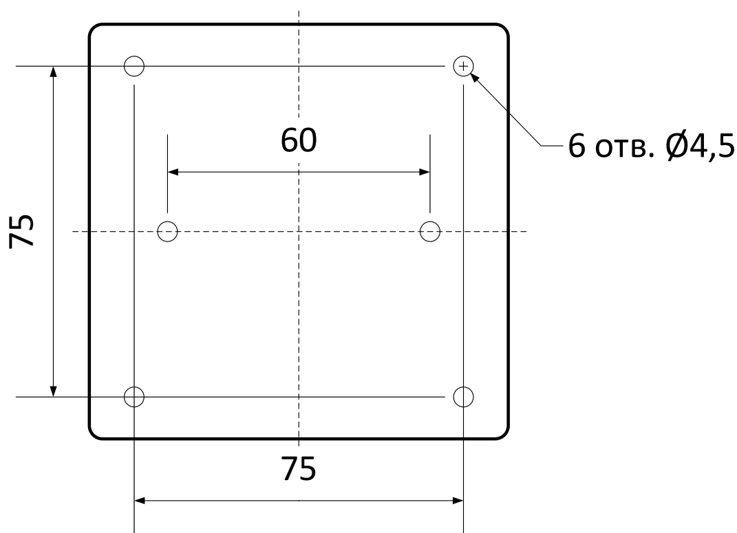
Рисунок 120 – Установочные размеры ИПР-И.
