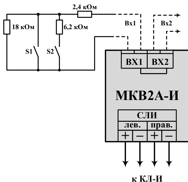
Рисунок 129 – Схема подключения внешних цепей к МКВ2А-И.
