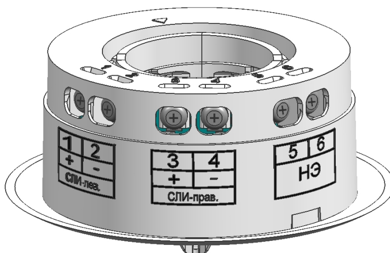
Рисунок 104 – Клеммы подключения внешних цепей к ИПТ-СИ-ку, ИПТ-СИ-кс, МКС-И-ку, МКС-И-кс.
