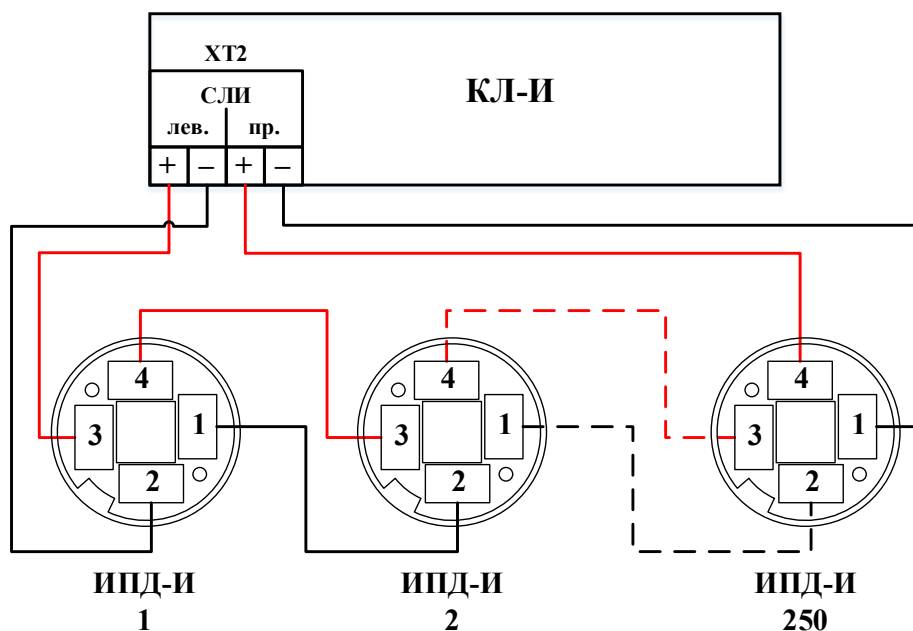
Рисунок 112 – Схема подключения ИПД-И к КЛ-И (КЛ-И-2).
