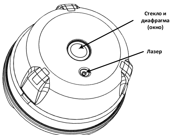
Рисунок 114 – Извещатель пламени.
