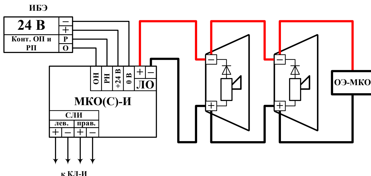
Рисунок 124 – Схема подключения оповещателей к МКО(С)-И.
