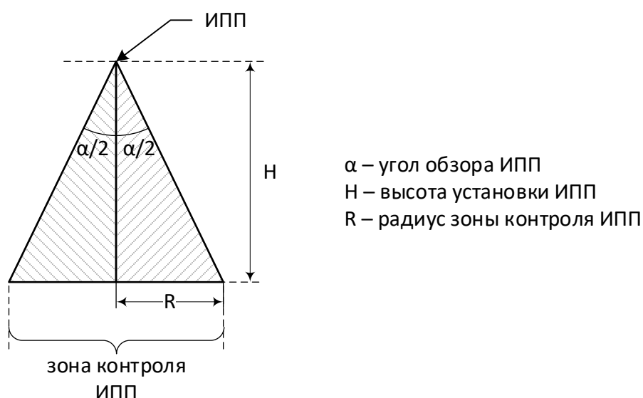
Рисунок 115 – Размер зоны контроля ИПП (вид сбоку).
