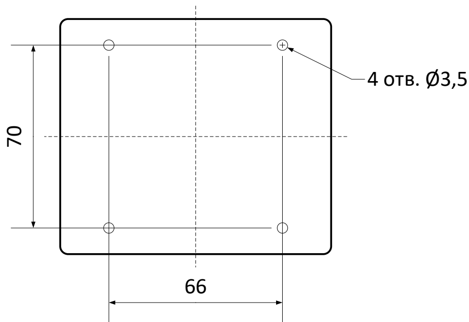
Рисунок 126 – Установочные размеры модулей МКО.
