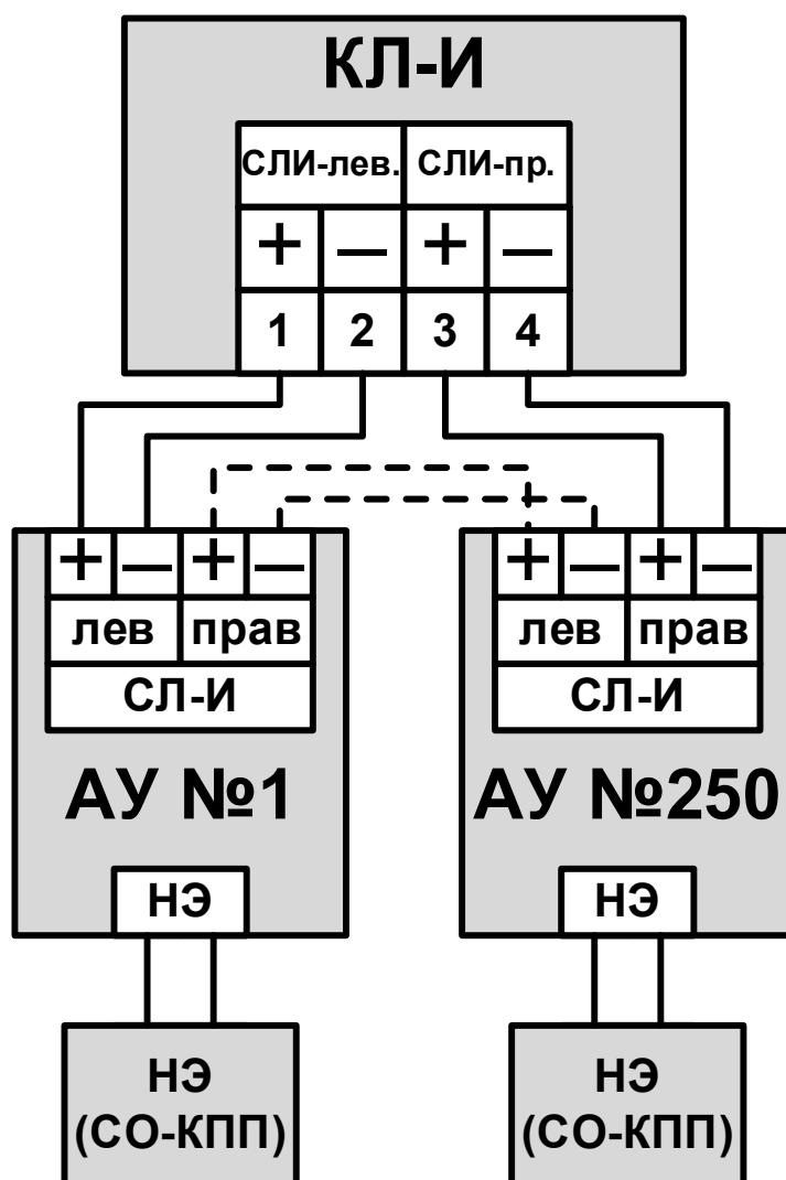
Рисунок 101 – Общая схема подключения АУ к КЛ-И (КЛ-И-2).
