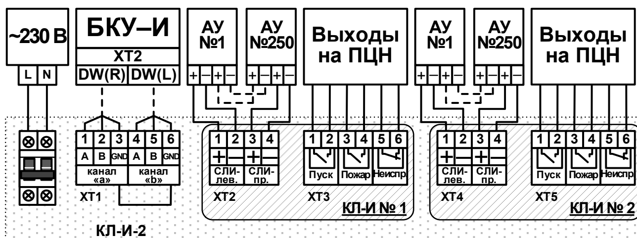
Рисунок 99 – Схема подключений КЛ-И-2.
