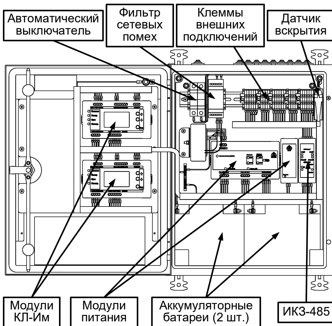
Рисунок 98 – Внешний вид КЛ-И-2 с открытой крышкой.
