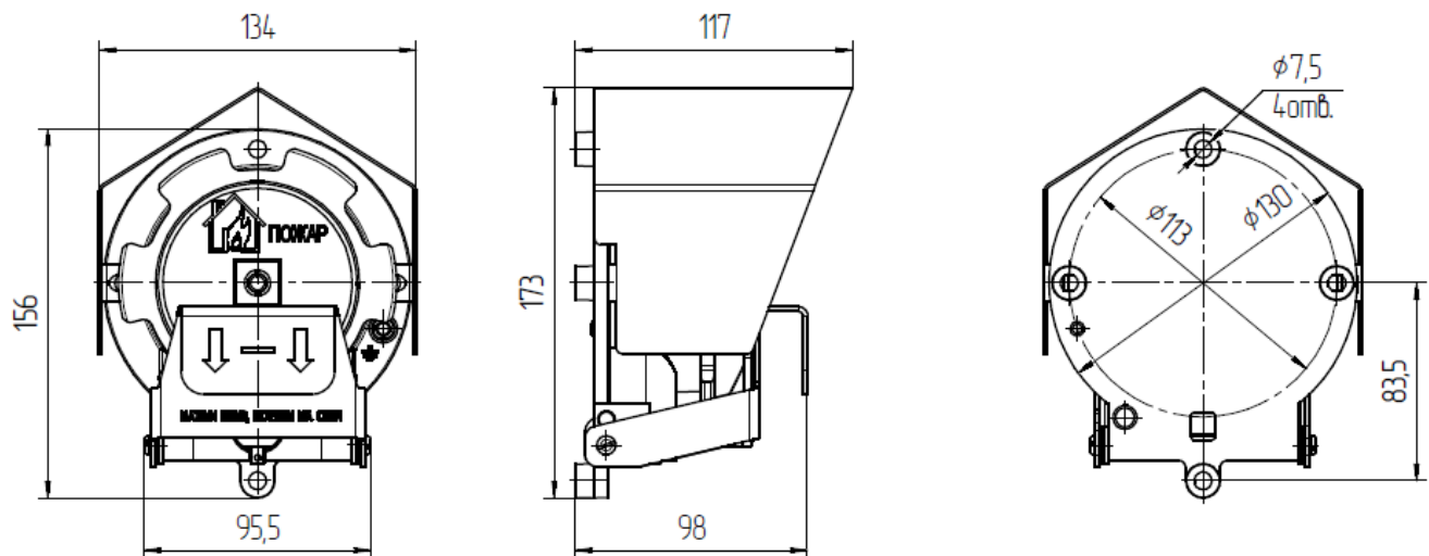
Рисунок А2 – Габаритные размеры «Спектрон-535-Exd-A-ИПР-В»
