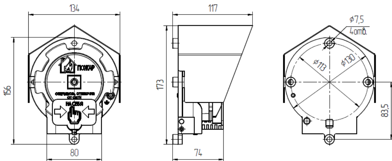
Рисунок А1 – Габаритные размеры извещателя «Спектрон-535-Exd-A-ИПР-A»
