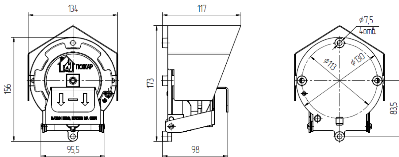
Рисунок А2 – Габаритные размеры «Спектрон-535-Exd-A-ИПР-B»
