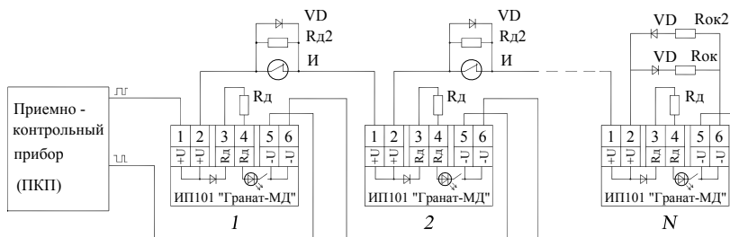
Рис.Б.2 Схема подключения извещателей ИП101 «Гранат-МД» в шлейф сигнализации со знакопеременным импульсным напряжением
