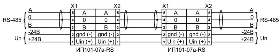
Рисунок 9. Схема подключения адресных извещателей ИП101-07а-RS к линии связи RS-485 с протоколом Modbus RTU с использованием комбинированного кабеля.
