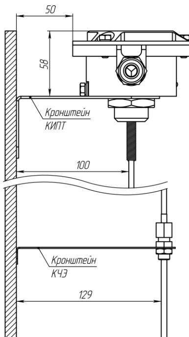
б) Крепление ИП1101-07мд-И2
