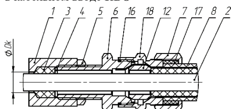
з) монтаж бронированным кабелем в кабельном вводе KBВУ
