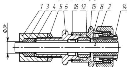
и) монтаж бронированным кабелем в металлорукаве в кабельном вводе KBВМ
