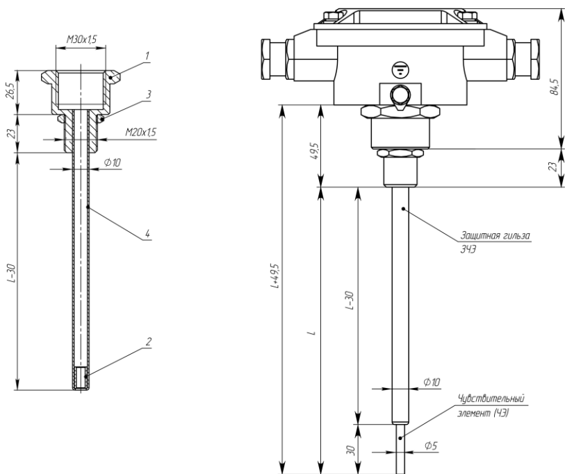
Рисунок 4. Монтаж защитной гильзы 3ЧЭ извещателя.
