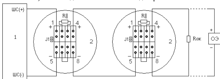
б) Схема подключения ИП101-07мд на замыкание
