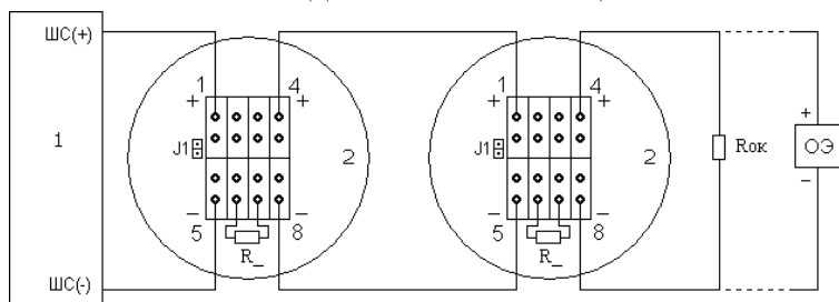
а) Схема подключения ИП101-07мд на размыкание
