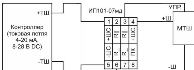
Рисунок 9. Схема подключения извещателя ИП101-07мд в линию типа “токковая петля 4-20 мА” с помощью МТШ.
