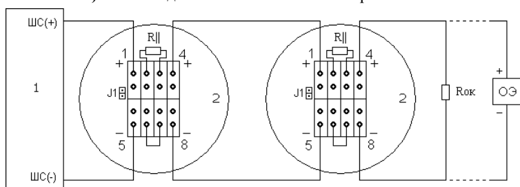
б) Схема подключения ИП101-07вт на замыкание
