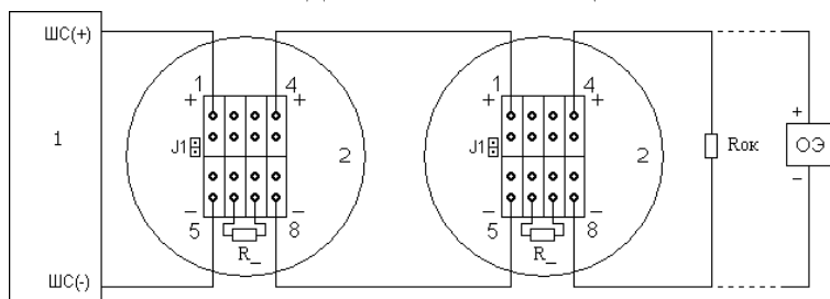
а) Схема подключения ИП101-07вт на размыкание
