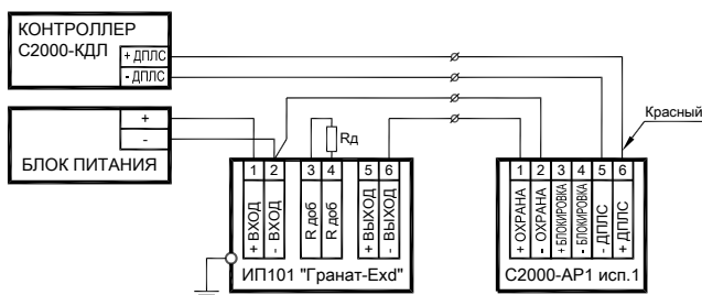
Рис.Б.1.2. Схема подключения адресного расширителя «С2000-AP1» исп.1 к извещателю ИП101 «Гарант-Exd»
