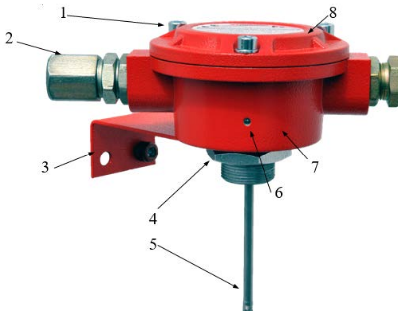
1 – винт M6 с шайбой; 2 – кабельный ввод; 3 – крепежное устройство (K-05); 4 – гайка M30x1,5; 5 – чувствительный элемент; 6 – светодиодный индикатор; 7 – корпус извещателя; 8 – крышка извещателя.
