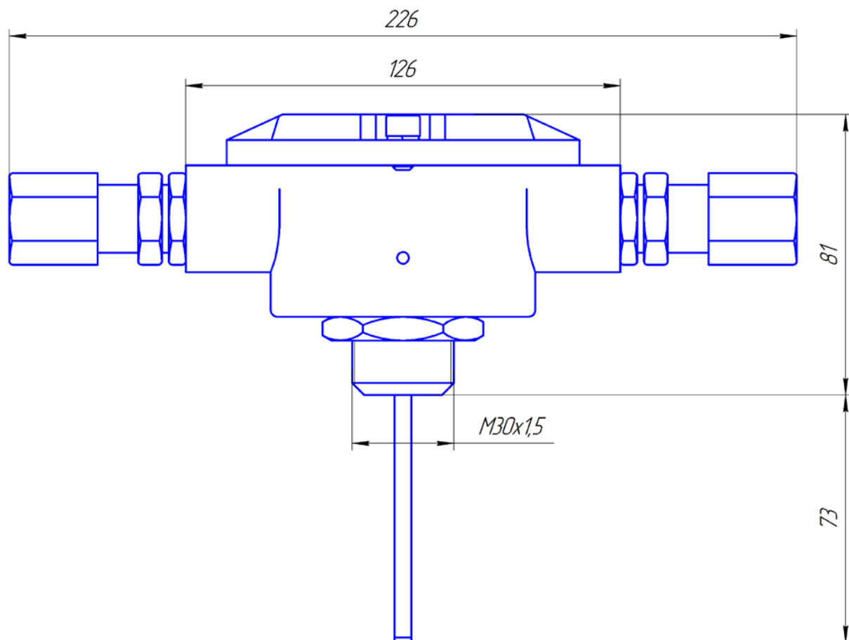
Рисунок А1 – Извещатель пожарный тепловой Спектрон-101-Р-Exd-A и Спектрон-101-Р-Exd-H
