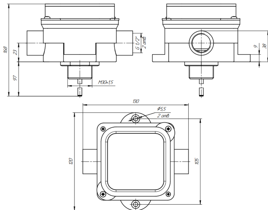
Рисунок А1. Габаритный чертеж на Спектрон-101-Р-Exi/Exm
