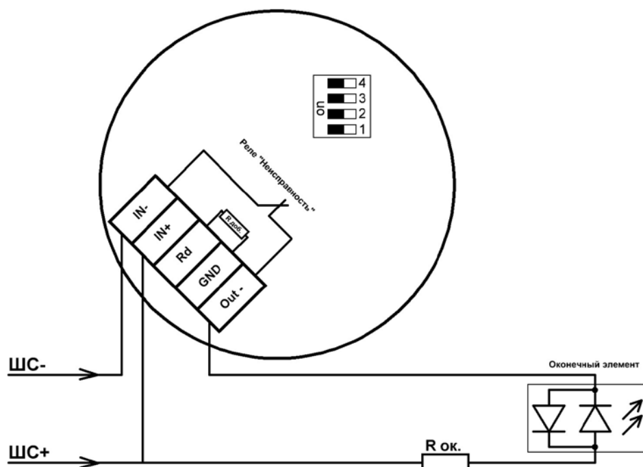
Рисунок Б1 – Подключения по 2-х проводной схеме с режимом «Неисправность»
