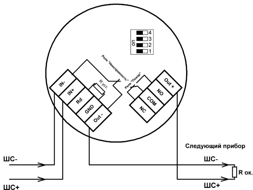
Рисунок Б1 – 2-х проводная схема подключения
