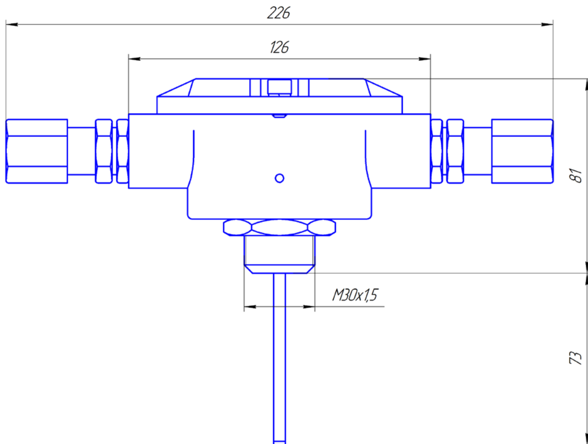
Рисунок А1 – Извещатель пожарный тепловой Спектрон-101-Т-Р-Exd-A и Спектрон-101-Т-Р-Exd-H
