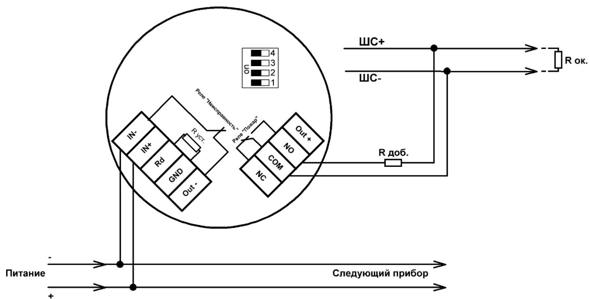
Рисунок Б2 – 4-х проводная схема подключения
