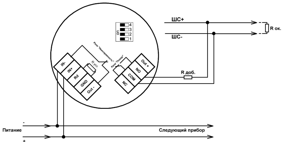
Рисунок Б2 – Подключение по 4-х проводной схеме
