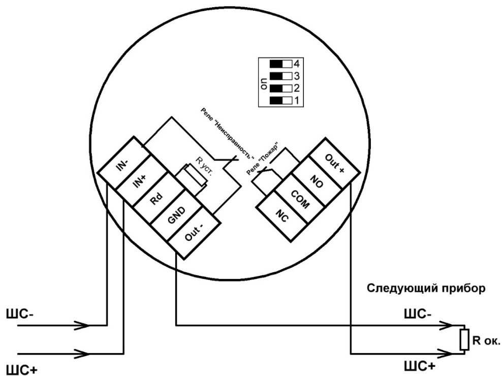
Рисунок Б1 – Подключения по 2-х проводной схеме
