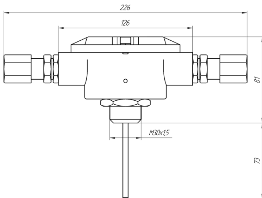
Рисунок А1.1 – Извещатель пожарный тепловой Спектрон-101-Т-Р-Exd-A/H-BЭ
