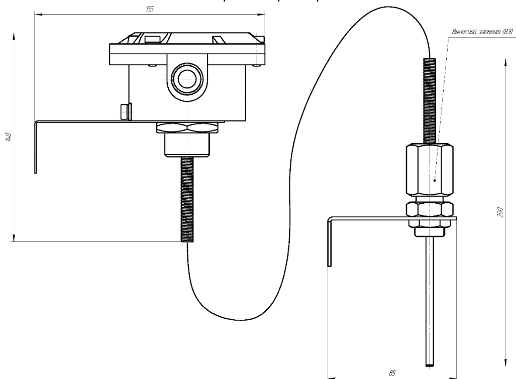
Рисунок А1 – Извещатель пожарный тепловой Спектрон-101-Т-Р-Exd-A/H-BЭ
