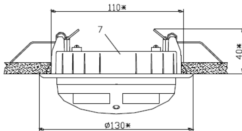
Рисунок 2.6 Монтажный комплект «МКЗ»
