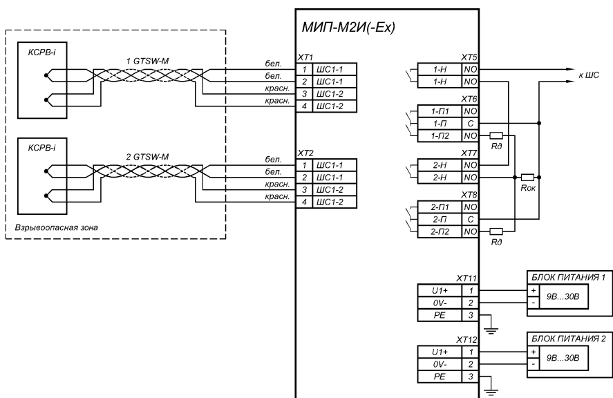
Рис. Г.2. Схема подключения модулей «МИП- М2И(-Ex)» для передачи извещений в один шлейф сигнализации.
