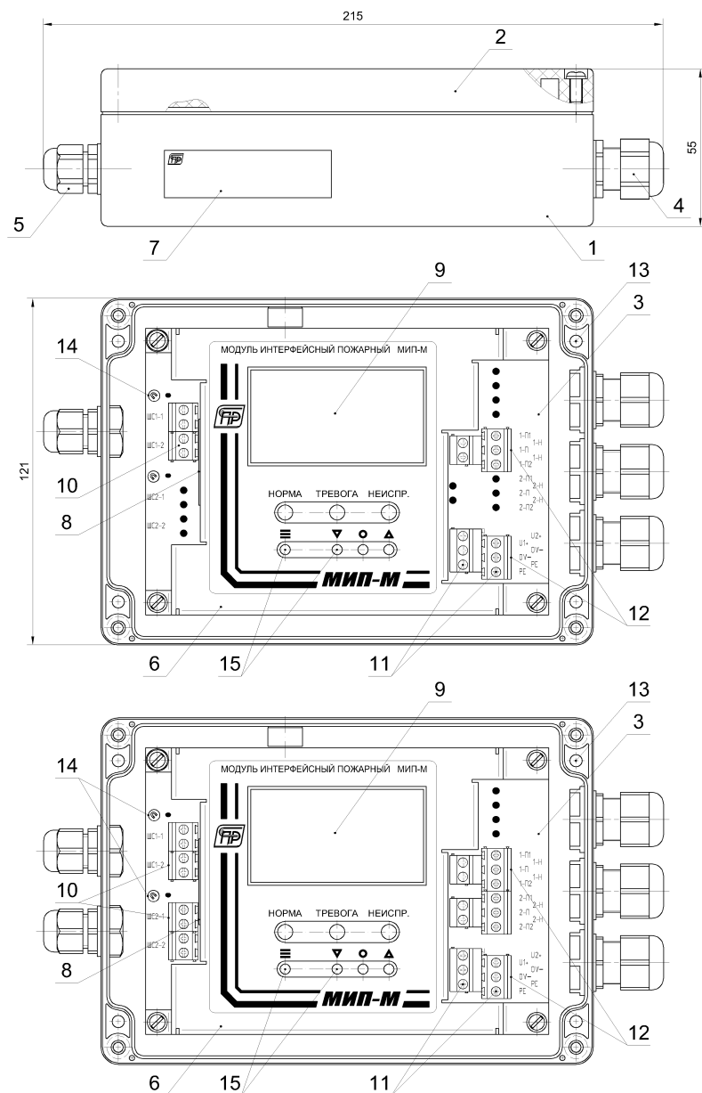
Рис. В.1. Внешний вид модулей МИП-М(1...2)И(-Ex).
