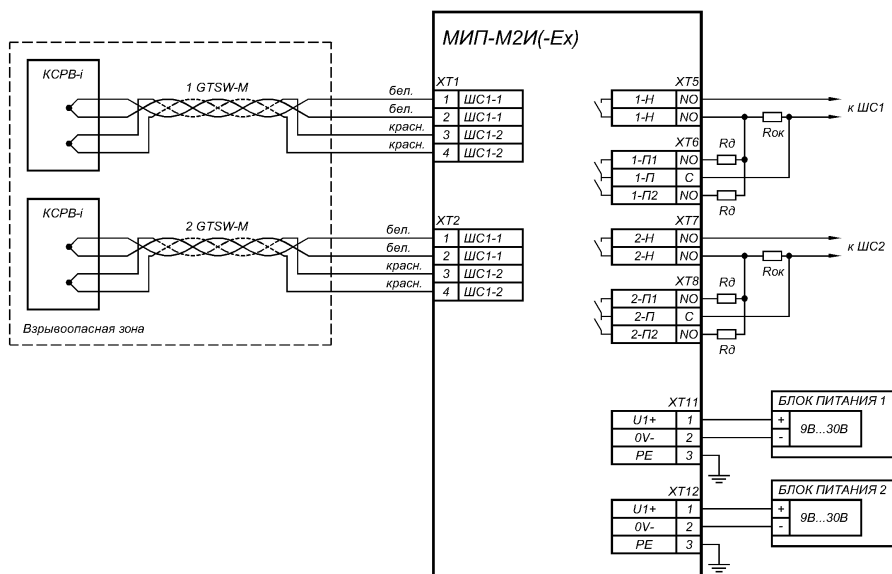
Рис. Г.1. Схема подключения модулей «МИП-М(1...2)И(-Ex)».
