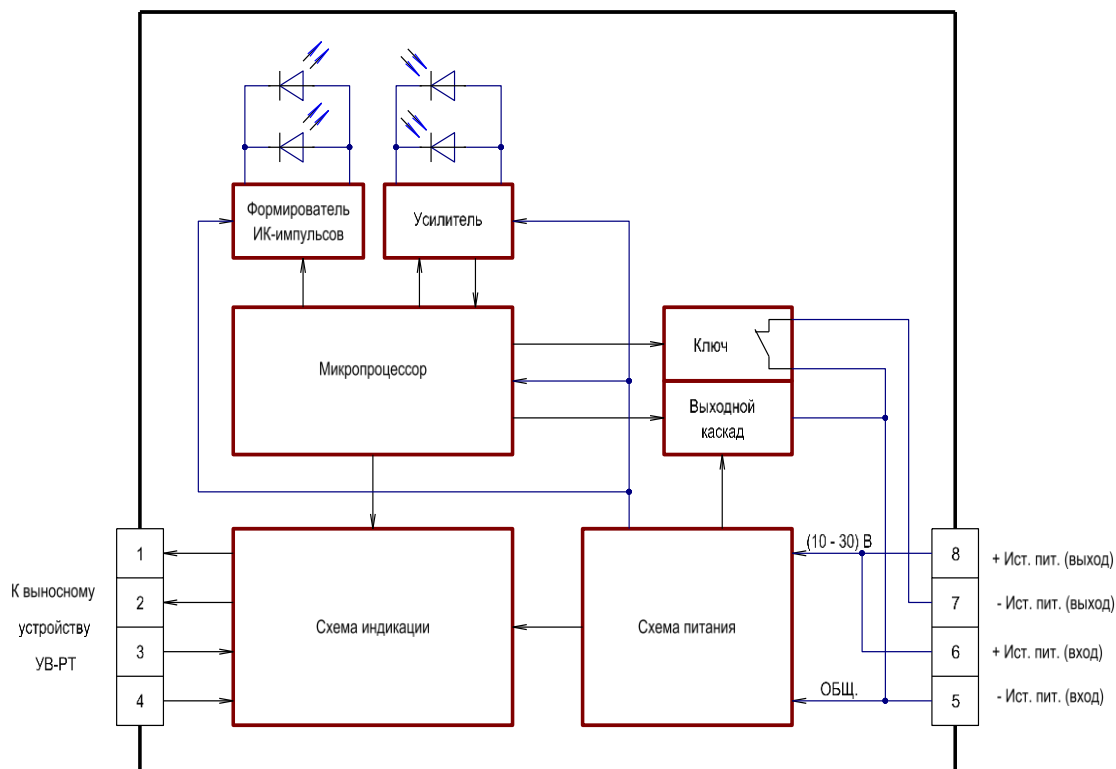
Рисунок 4. Структурная схема приёмо-передатчика
