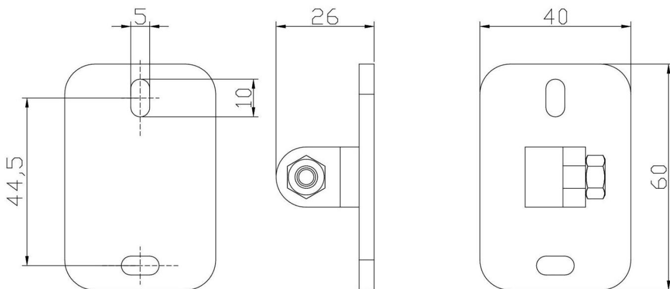
Рисунок 2.2.2.5 – Габаритные и установочные размеры крепления извещателя «С2000-Спектрон-608».
