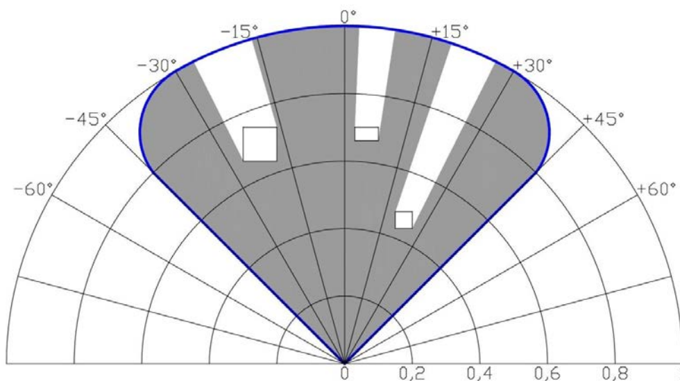
Рисунок 2.1.2.3 – Влияние посторонних предметов на зону чувствительности извещателя.
