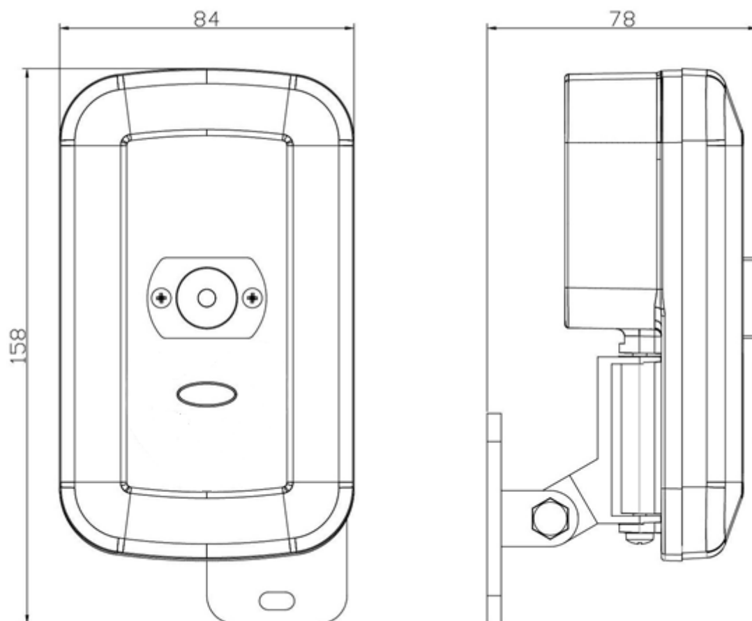
Рисунок 2.2.2.4 – Габаритные размеры извещателя «С2000-Спектрон-608».
