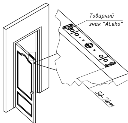
Рисунок 3 – Установка замка в горизонтальном варианте
