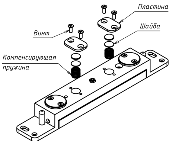
Рисунок 4 – Демонтаж пружин якоря для вертикального варианта замка
