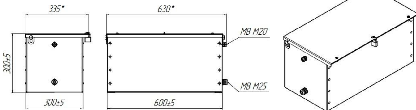
Рис.1 Габаритные размеры Бокса под АКБ.
