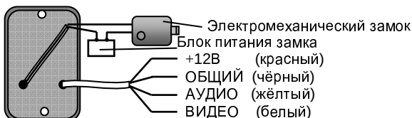
Схема подключения панели JSB-V081
