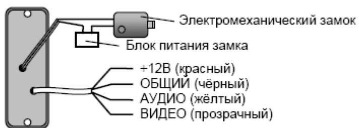
Схема подключения панели JSB
