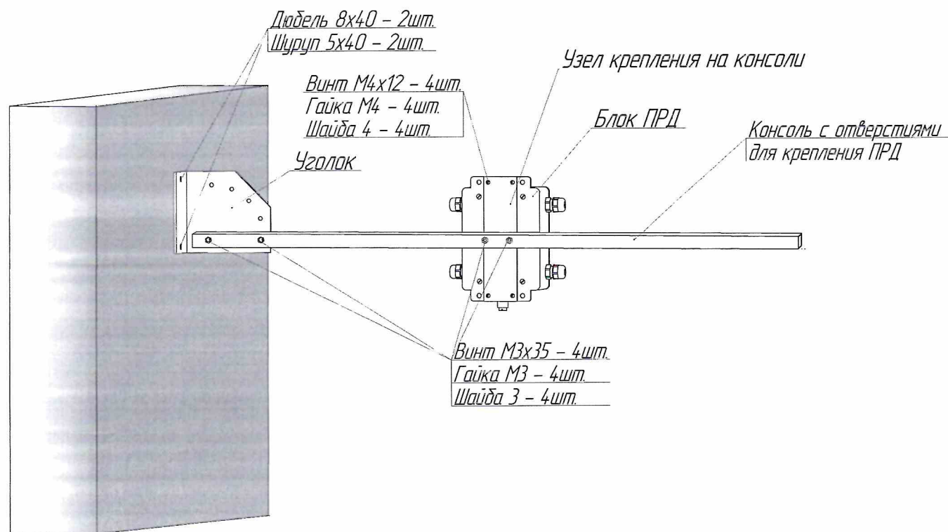
Рисунок 2.4 – Установка ПРД на консоли
