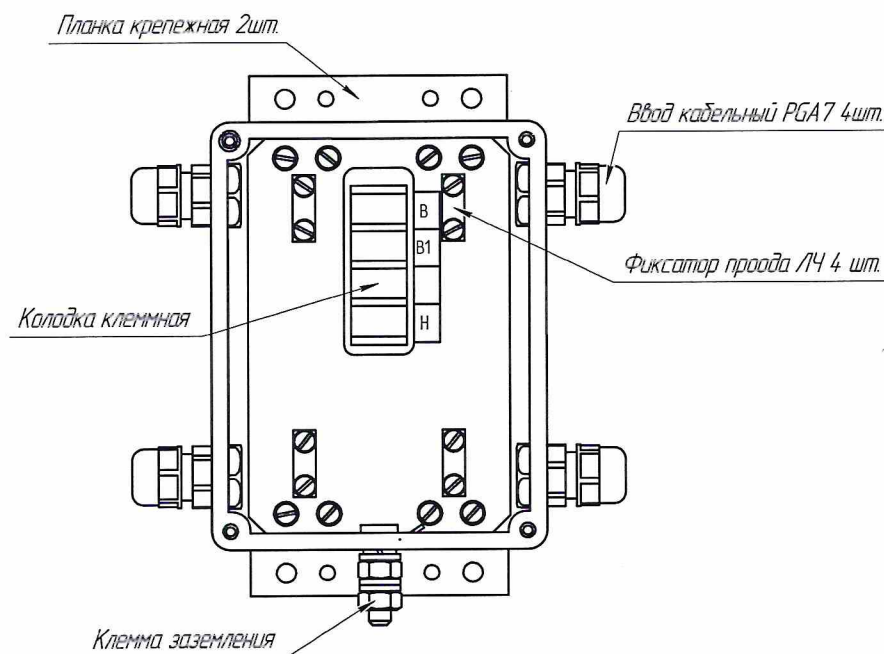
Рисунок 1.2 – Блок ПРД со снятой крышкой
