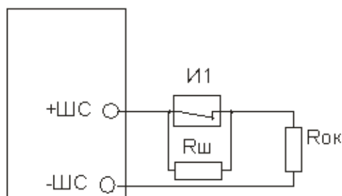
Рисунок 12 – Охранный ШС
