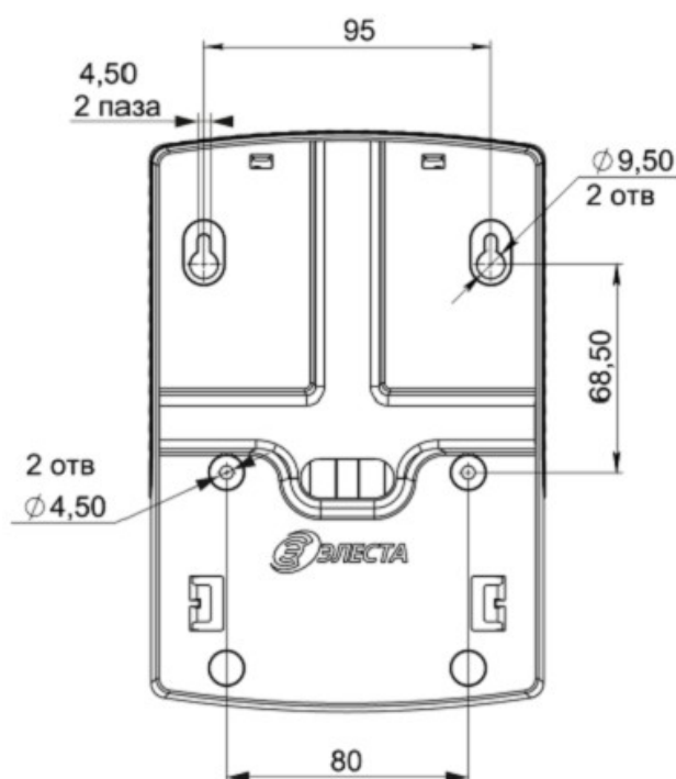
Рисунок 2. Установочные размеры прибора
