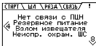
Рисунок 12 – Экран тревожных сообщений и неисправности «!».
