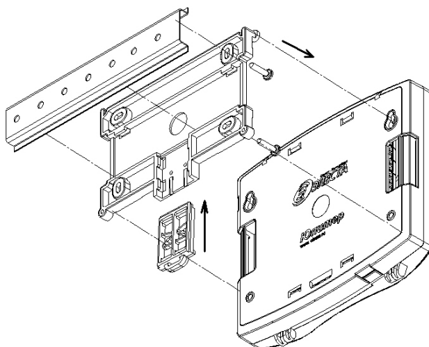
Рисунок 17 – Вариант установки прибора через переходную планку на DIN-рейку (вид с задней крышки прибора)
