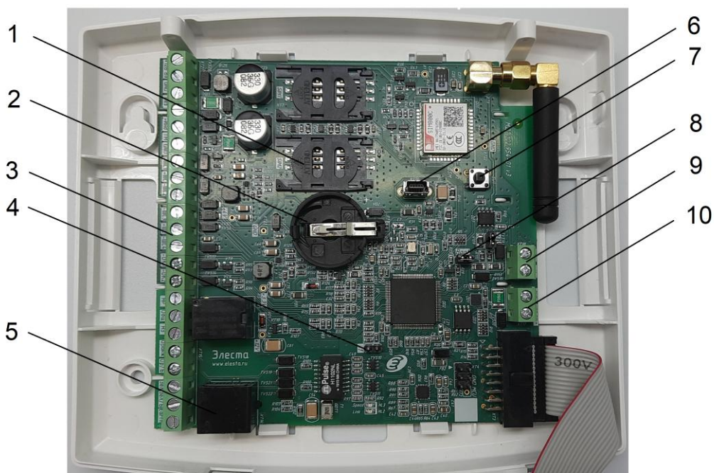
Рисунок 3 – Вид основной платы прибора
