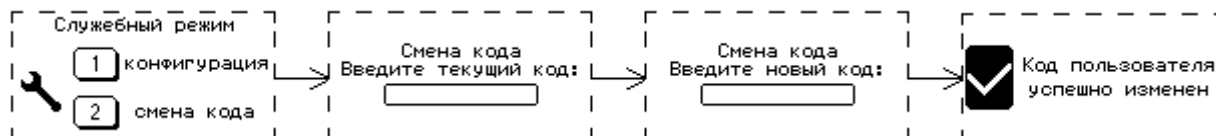
Рисунок 22 – Изменение кода пользователя в приборе Юпитер-2444
