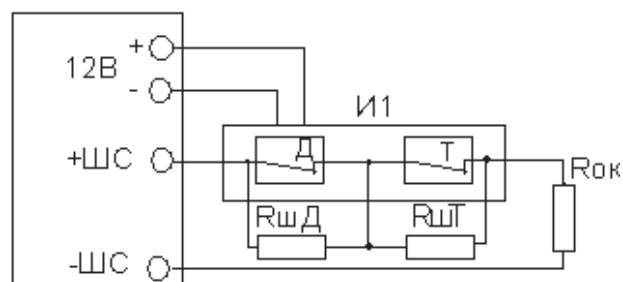
Рисунок 20 – ШС охранный с контролем взлома извещателей, с внешним питанием
