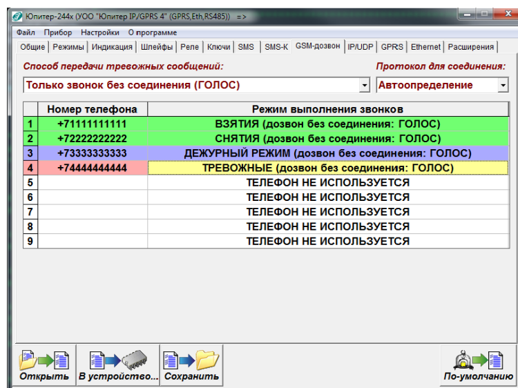
Рисунок 13 – Настройка номеров дозвона без соединения
