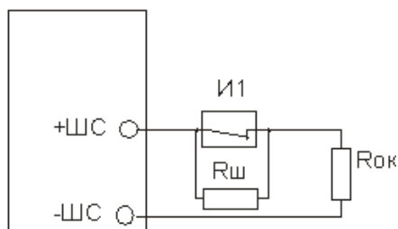
Рисунок 18 – ШС охранный
