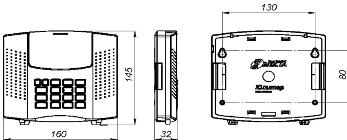
Рисунок 15 – Габаритные и установочные размеры прибора
