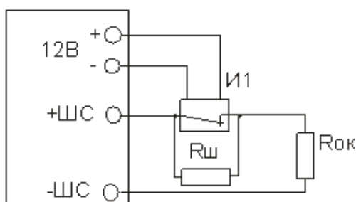
Рисунок 19 – ШС охранный с внешним питанием
