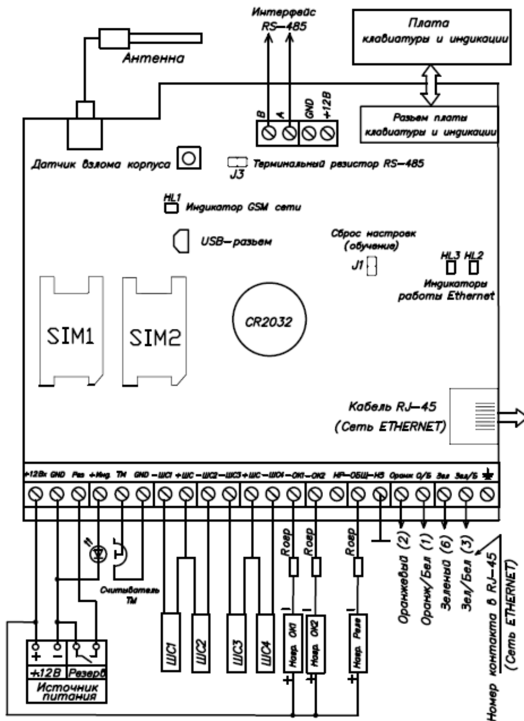
Рисунок 7 – Назначение разъемов УОО «Юпитер-24xx»
