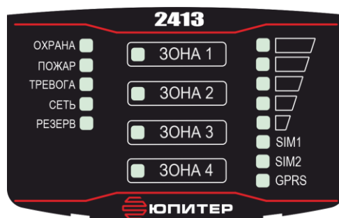
Рисунок 4 – Панель индикации УОО в исполнении Юпитер-2413
