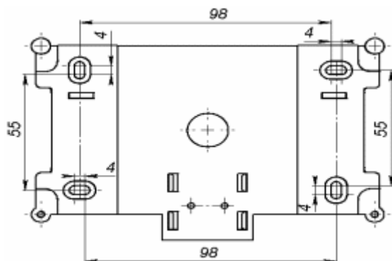
Рисунок 16 – Габаритные размеры переходной планки
