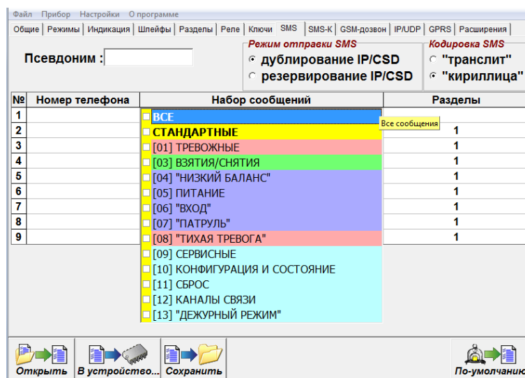
Рисунок 14 – Настройка набора событий, передаваемых с помощью СМС-сообщений.
