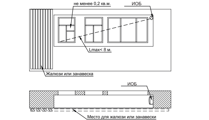
Рисунок 3а Установка ИОБ в оконном проеме
