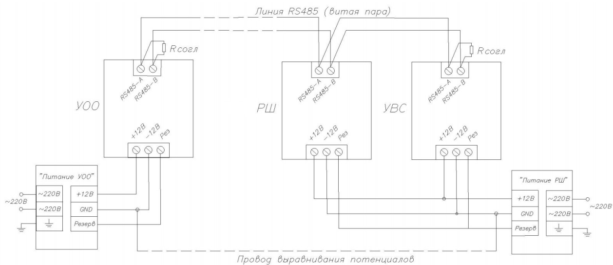
Рисунок 4.4. Пример схемы подключения YBC и расширителя по линии RS485
