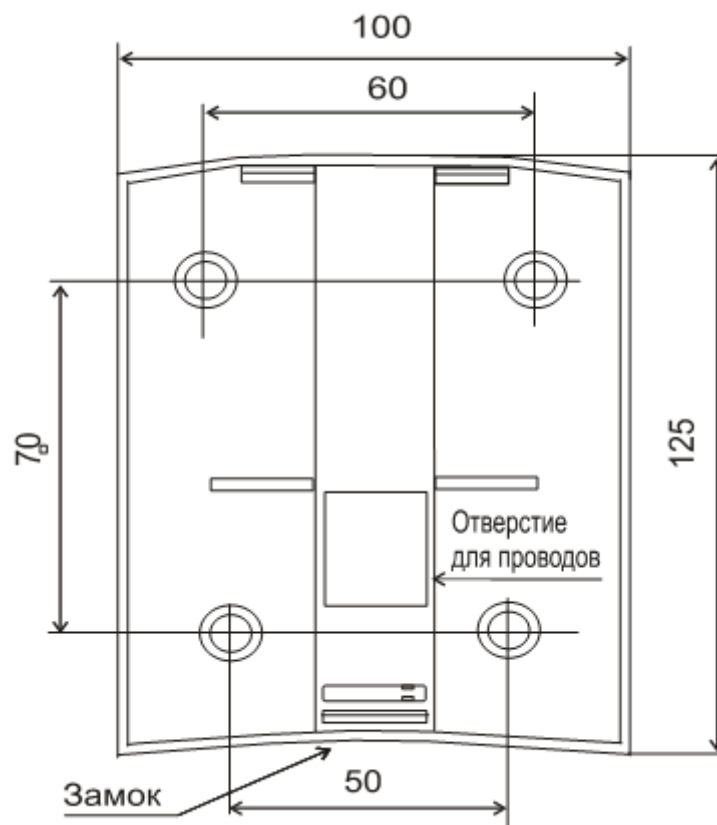
Рисунок 4.1. Габаритные и установочные размеры прибора
