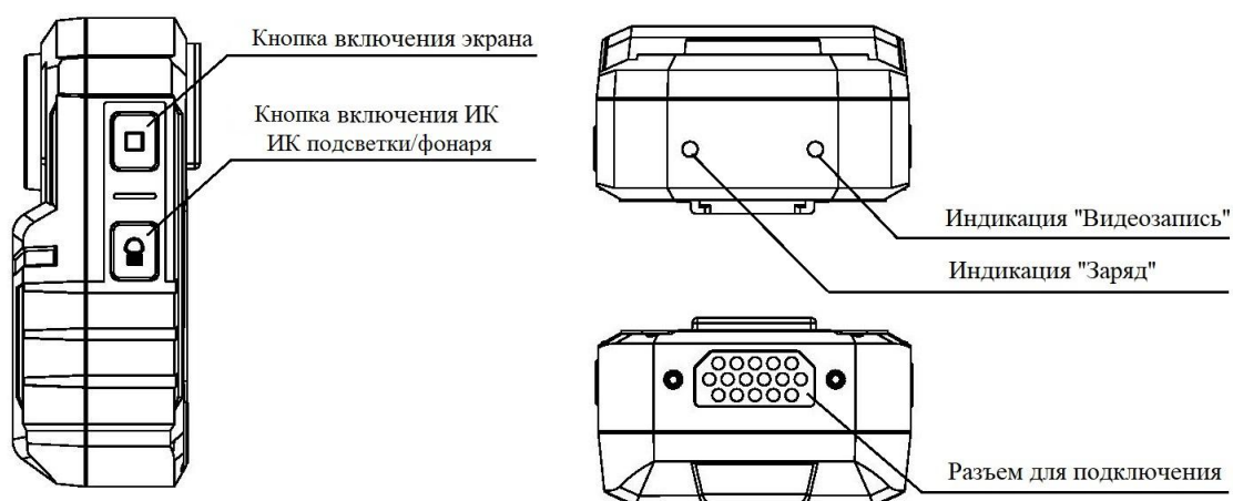
Рисунок 2 – Внешний вид видеорегистратора «Юпитер-7412».
