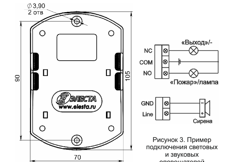
Рисунок 2. Установочные размеры «Ю-7620»
