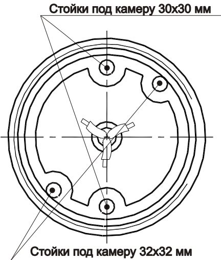
Рис.2 Вид сзади гермокожуха
