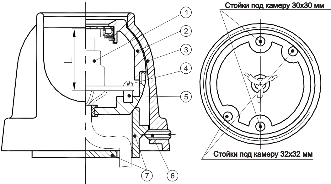
Рис.1 Устройство гермокожуха
