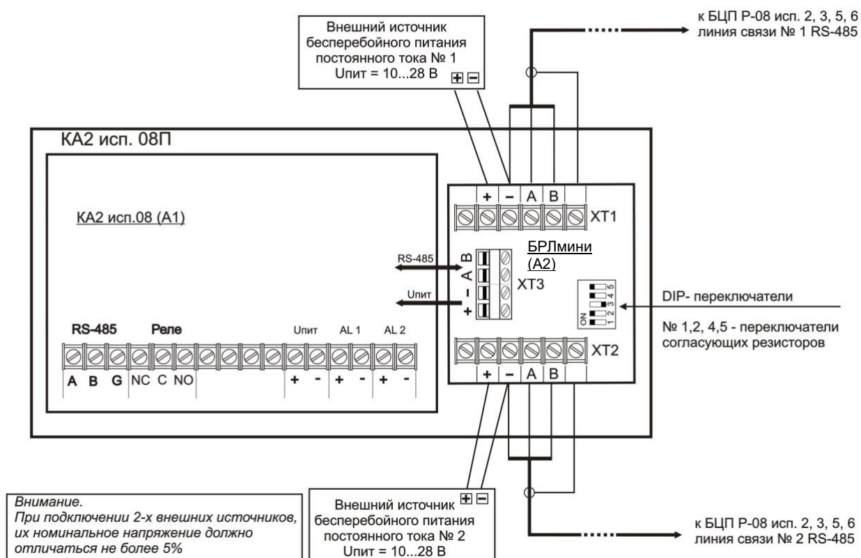
Рис. 3 Применение (подключение) КА2 исп.08П
