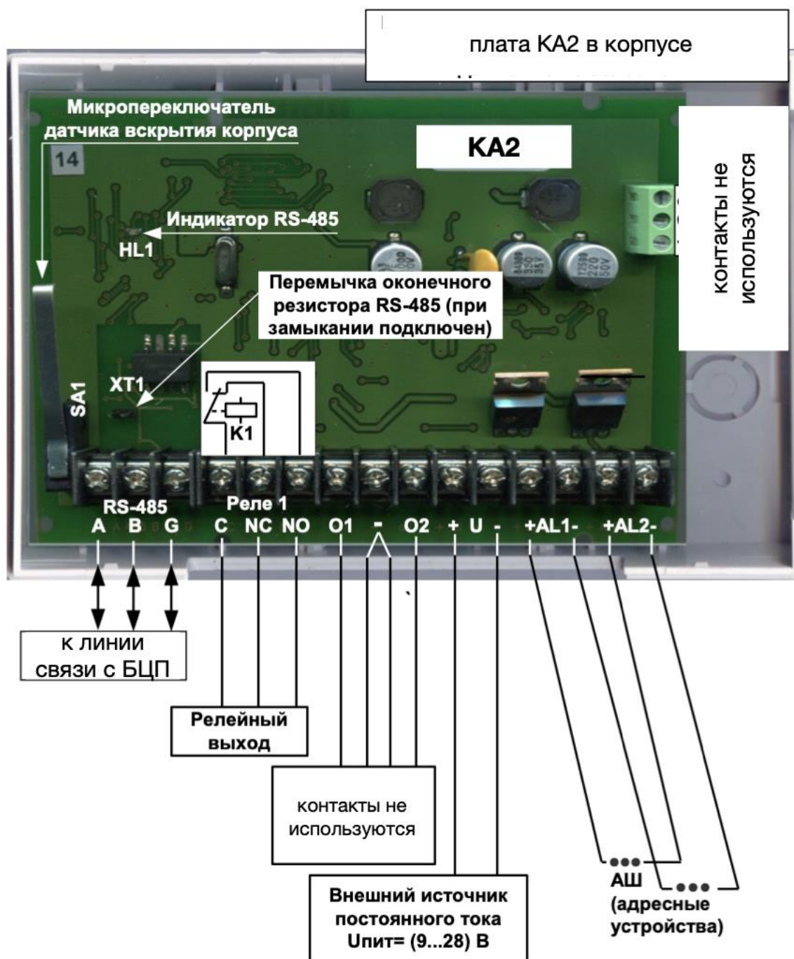
Рис. 1 Внешний вид KA2. Клеммы подключения.
