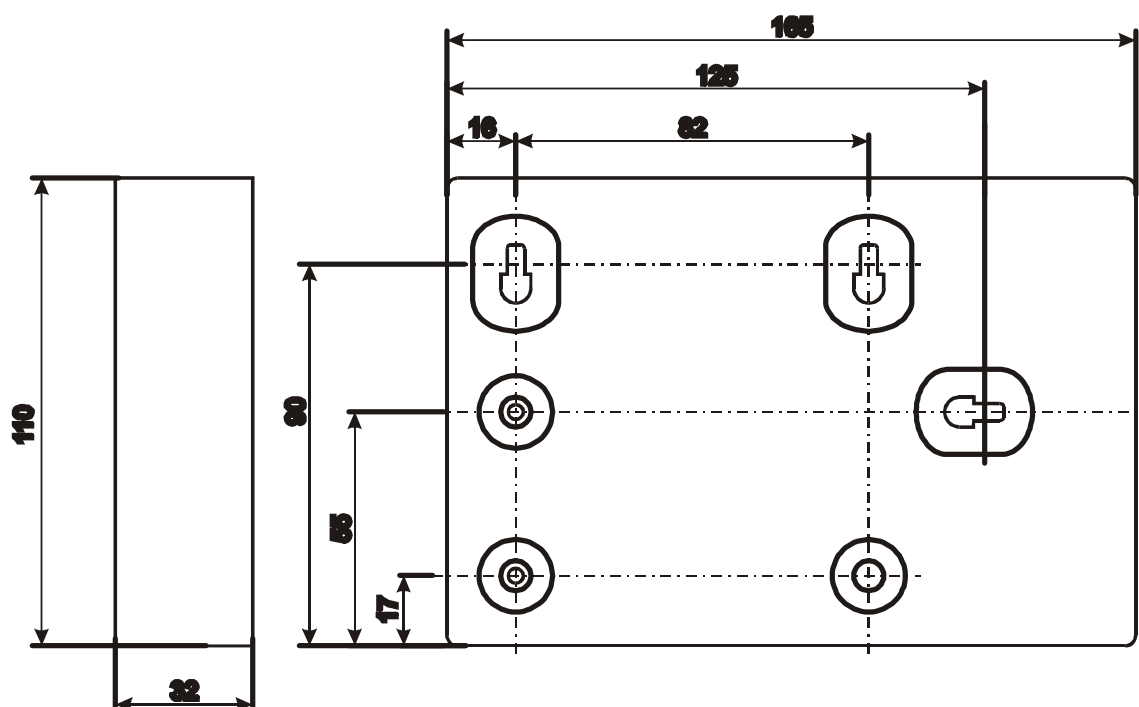
Рис. 2 Габаритные и присоединительные размеры КА2 исп. IP20
