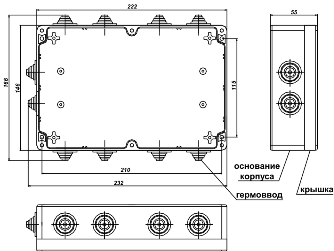
Рис. 4 Габаритные и присоединительные размеры КА2 исп.08П
