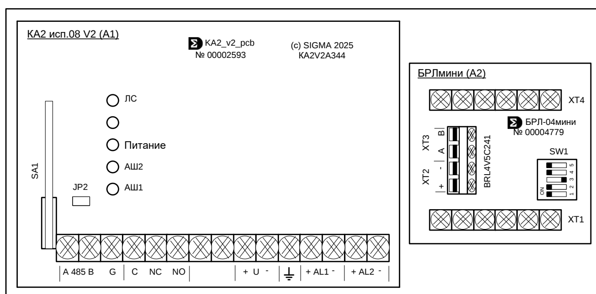
Рис. 7 Клеммы подключения КА2 исп.08П V2
