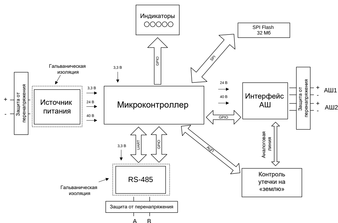
Рис. 2 Функциональная блок-схема КА2 исп.08 V2
