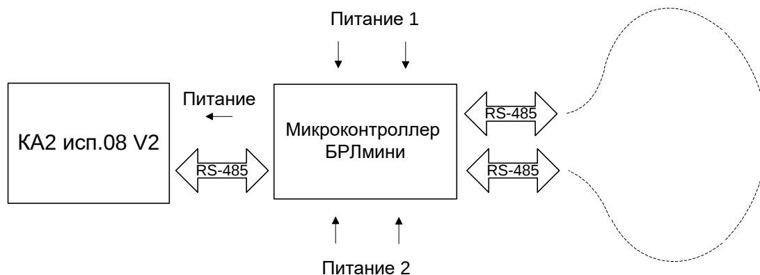
Рис. 3 Функциональная блок-схема КА2 исп.08П V2
