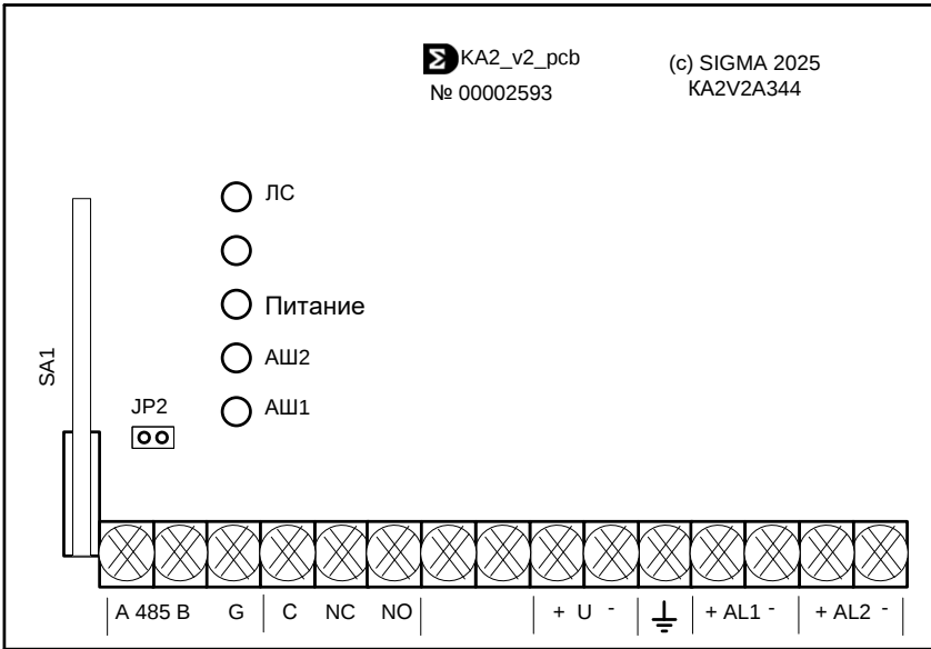
Рис. 6 Клеммы подключения КА2 исп.08 V2
