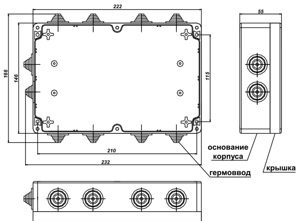
Рис. 5 Габаритные размеры КА2 исп.08П V2
