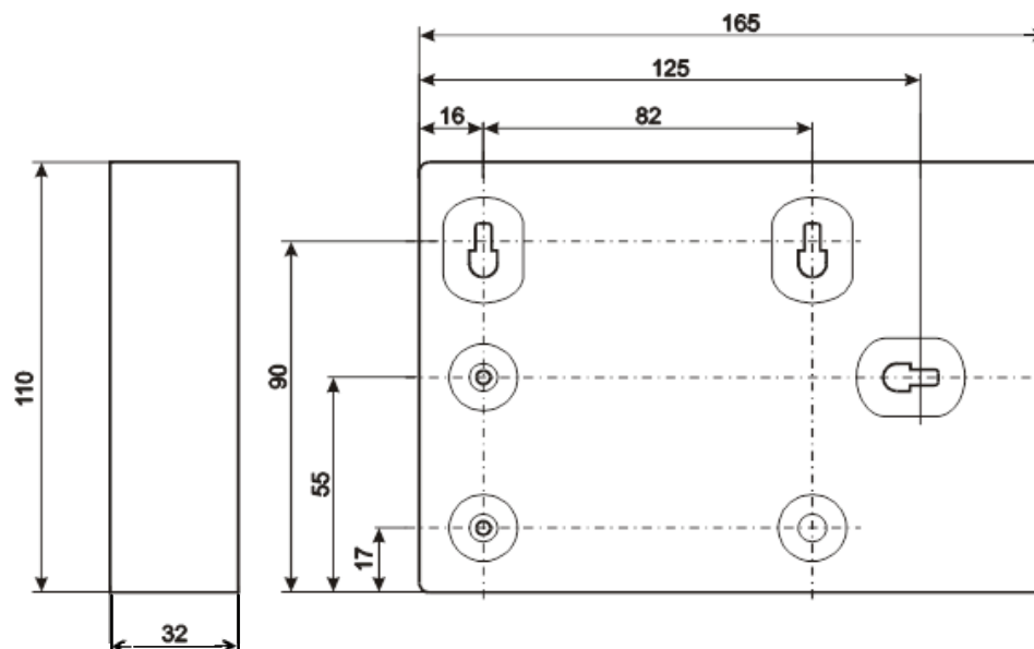
Рис. 4 Габаритные и присоединительные размеры КА2 исп.08 V2
