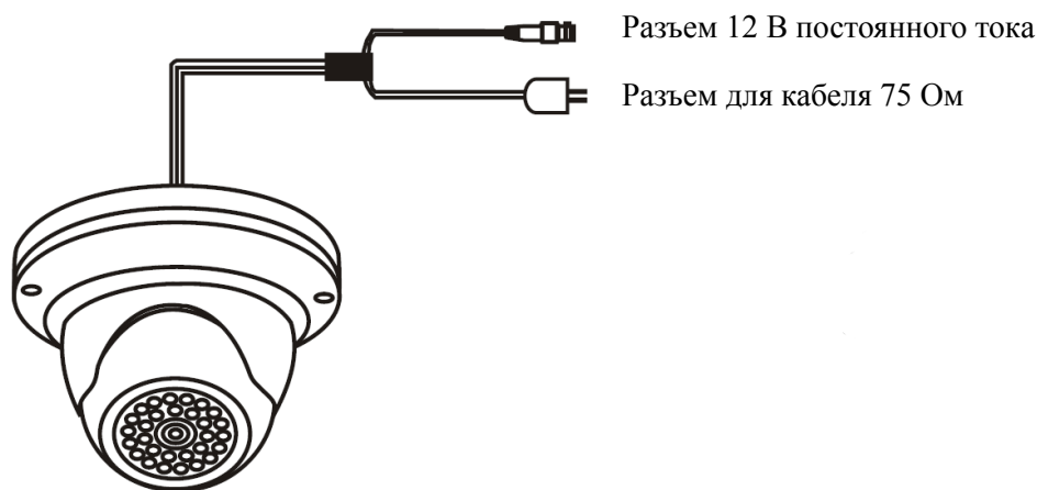
Рисунок 3.1 Разъемы
