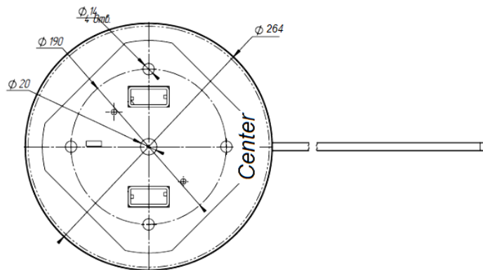
Рисунок 4- Установочные размеры площадки
